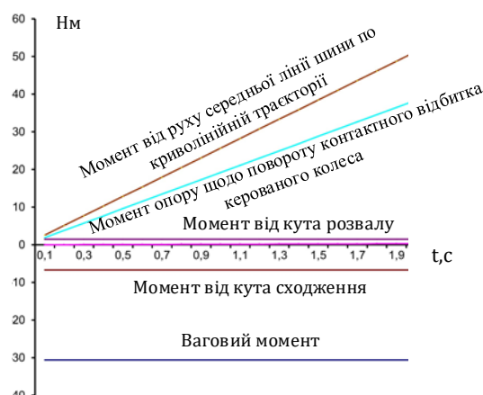
Рис. 1. Моменти діючі в плямі контакту керованого колеса з опорною поверхнею
