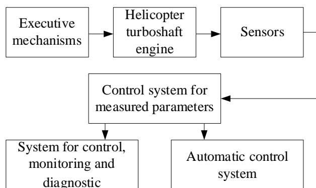
Рис. 1. Структура цифрової системи управління ГТД вертольотів
