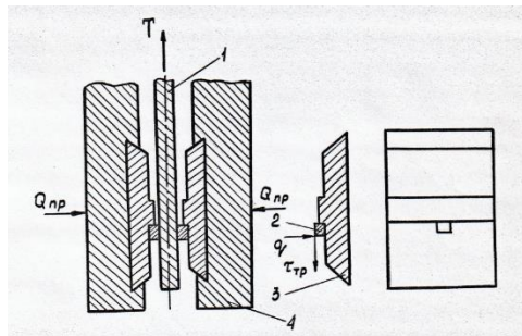
Рис. Вузол тертя пластинчатої машини тертя
